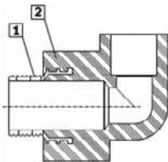
Рисунок 10. Комбинированный фитинг
