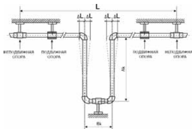
Рисунок 3. П-образный компенсатор
