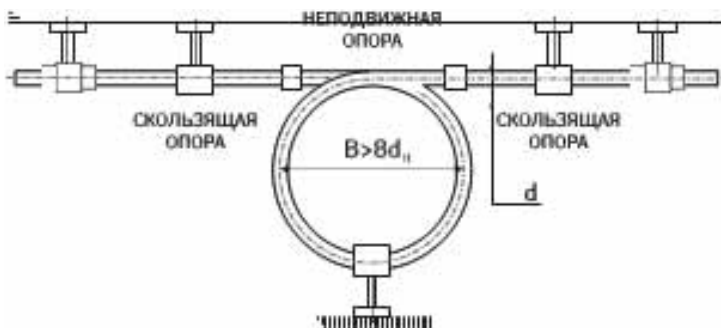
Рисунок 5. Петлевой компенсатор
