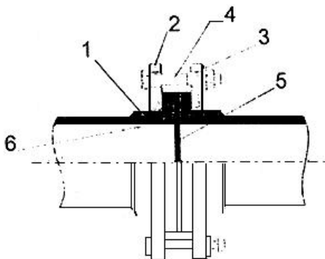
Рис.5.3. Соединение труб из PPRC на свободных фланцах
