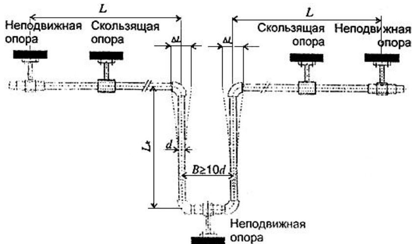
Рис.2.5. П-образный компенсатор
