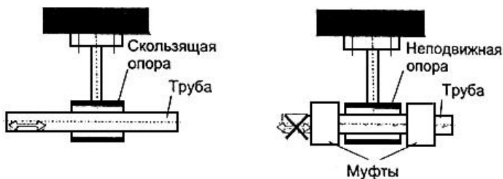
Рис.4.1. Виды опор
