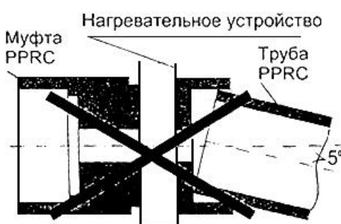
Рис.5.2. Технологическая операция "нагрев"
